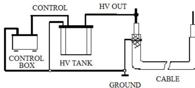
Figura 8. Medición del diagrama de conexión monofásica.
